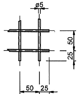
dettaglio A scala 1 : 5
